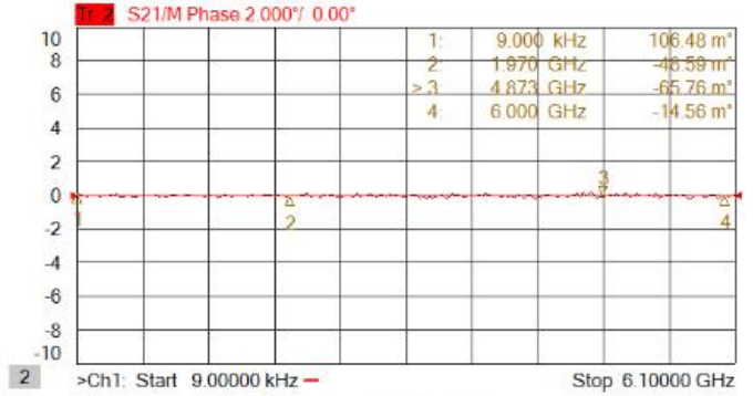
图2.相位平衡
