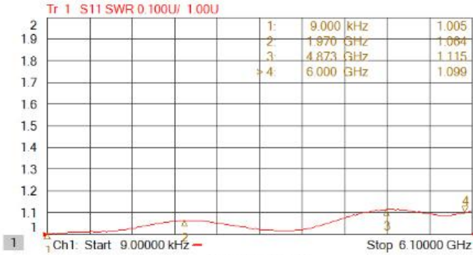
图1.合路端驻波比
