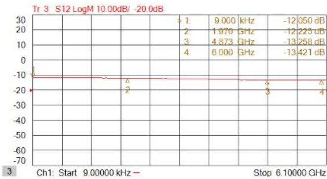
图3.插入损耗
